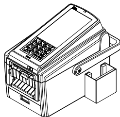
スキャナーホルダー 取付け後の全体図
